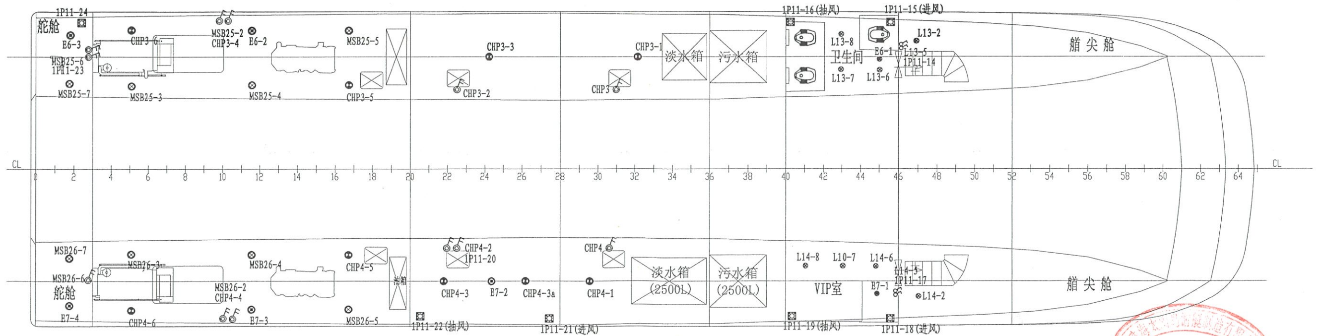
舱底布置图
