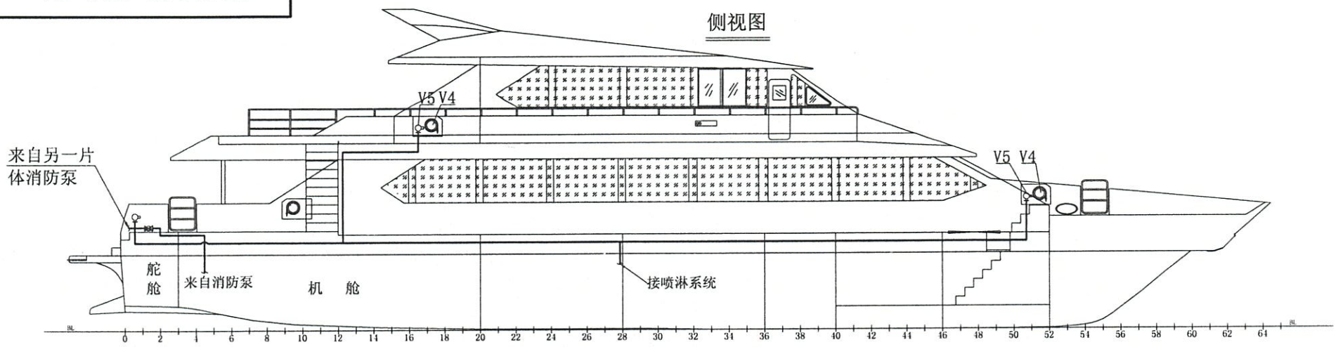
上甲板舱室布置图
